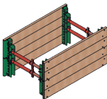
KRINGS Flex-Verbau empf. Verbautiefe bis 2,00 m empf.: Minibagger 3–9 t Seite 189
