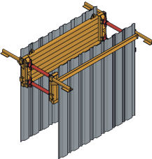
KRINGS BLU 2,41 m empf. Verbautiefe bis 2,40 m empf.: Mobilbagger 9–13 t Seite 182
