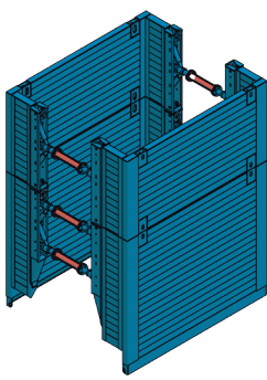
E+S Manhole empf. Verbautiefe bis 4,00 m empf.: Mobil- oder Kettenbagger 18–30 t Seite 172
