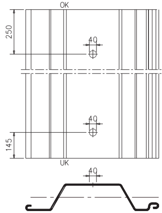
Die Leichtprofile FLP werden gelocht geliefert. Die Lochung erfolgt gemäß Abbildung an beiden Enden.
