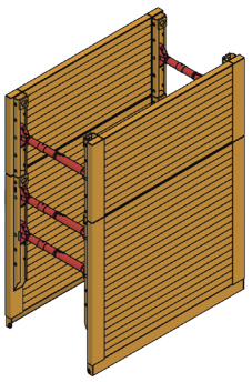
KRINGS KS 100 empf. Verbautiefe bis 4,00 m empf.: Mobil- oder Kettenbagger nur Grundbox: 12–18 t mit Aufsatzbox: 18–30 t Seite 168
