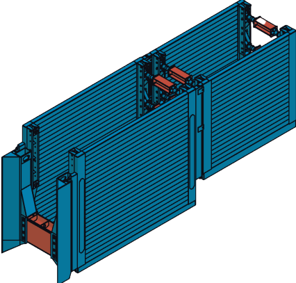
E+S Dragbox empf. Verbautiefe bis 5,00 m empf. Kettenbagger 30–50 t Seite 180
