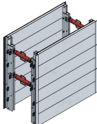
Alu-Leichtverbau empf. Verbautiefe bis 3,00 m empf.: Minibagger 3–9 t Seite 190
