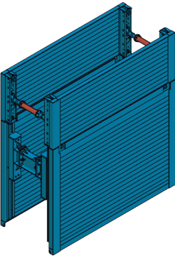
E+S Linearbox empf. Verbautiefe bis 5,00 m empf.: Mobil- oder Kettenbagger 18–30 t Seite 174
