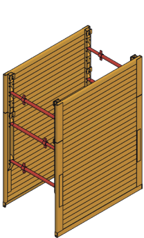
KRINGS KVL empf. Verbautiefe bis 3,50 m empf.: Mobilbagger 9–13 t Seite 158
