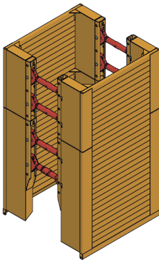
KRINGS KS 60 Eck empf. Verbautiefe bis 3,50 m empf.: Mobil- oder Kettenbagger nur Grundbox: 12–18 t mit Aufsatzbox: 18–30 t Seite 164
