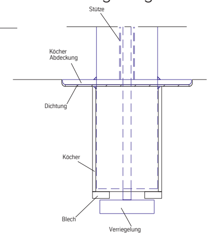
Ansicht Köcher mit Verriegelung
