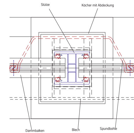
Ansicht Köcher mit Verriegelung
