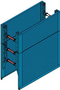
E+S Medium empf. Verbautiefe bis 5,00 m empf.: Mobil- oder Kettenbagger nur Grundbox: 12–18 t mit Aufsatzbox: 18–30 t Seite 166
