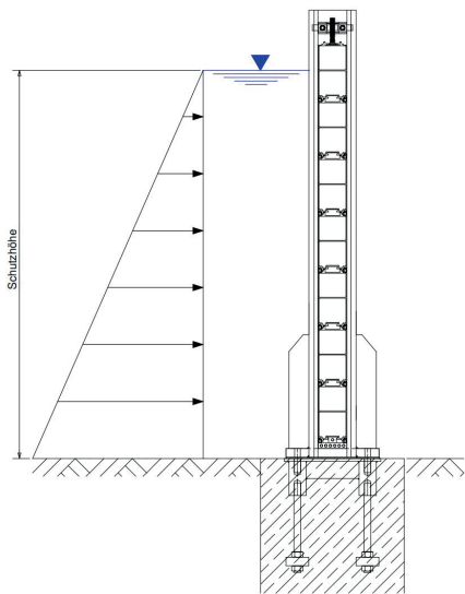
Belastungsfall 1: Wasserdruck
