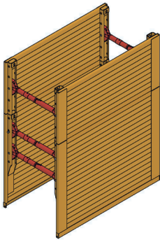
KRINGS KS 60 empf. Verbautiefe bis 3,50 m empf.: Mobil- oder Kettenbagger nur Grundbox: 12–18 t mit Aufsatzbox: 18–30 t Seite 162
