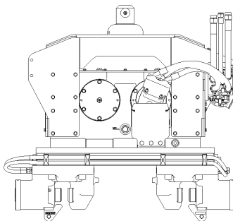
Abbildung zeigt MS-9 HFB mit Rohrkonsol DA 1160
