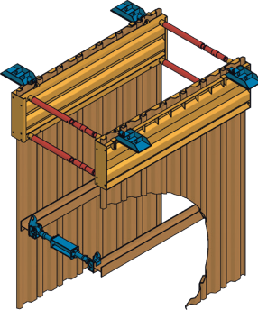
KRINGS DKU 2,27 m/3,00 m/3,81 m empf. Verbautiefe variabel empf.: Mobil- oder Kettenbagger 12–18 t Seite 184
