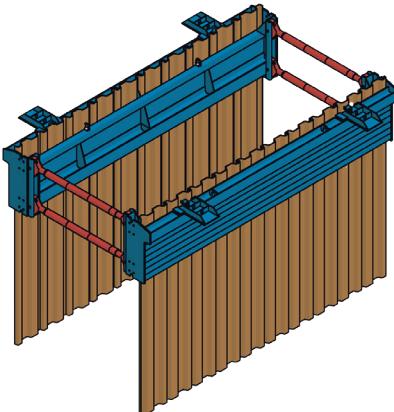
KRINGS DKU 4,55 m/5,80 m empf. Verbautiefe variabel empf.: Mobil- oder Kettenbagger 18–30 t Seite 186
