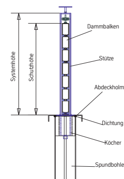
Querschnitt A-A
