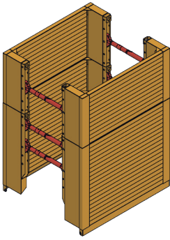
KRINGS KS 100 Eck empf. Verbautiefe bis 4,00 m empf.: Mobil- oder Kettenbagger 18–30 t Seite 170
